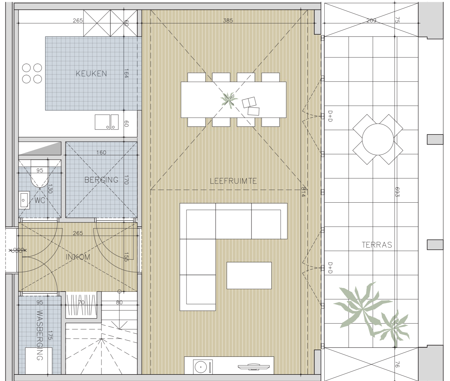
PLAN TOEGANG WONING - NIVEAU +1
