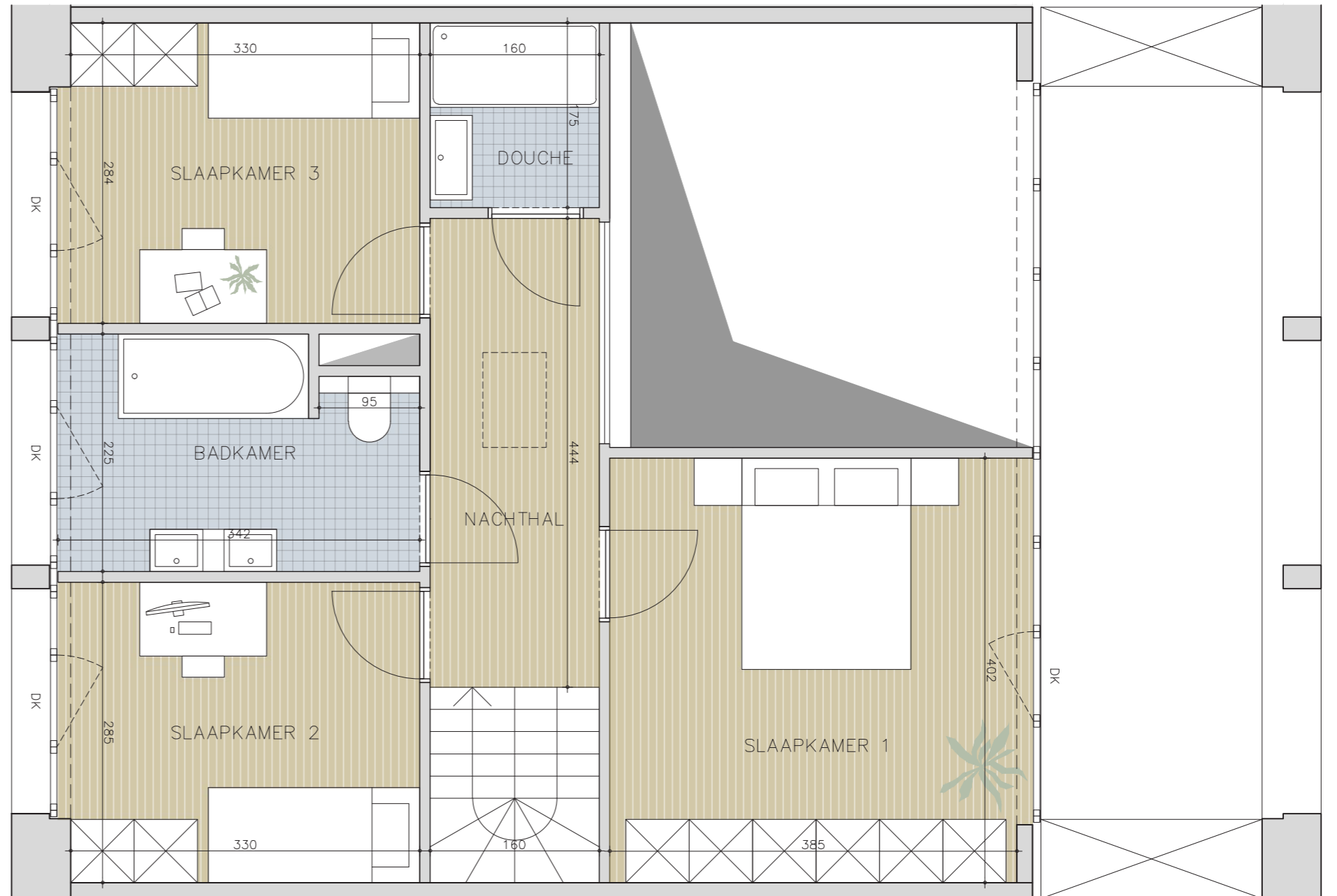
PLAN VERDIEPING - NIVEAU +2
