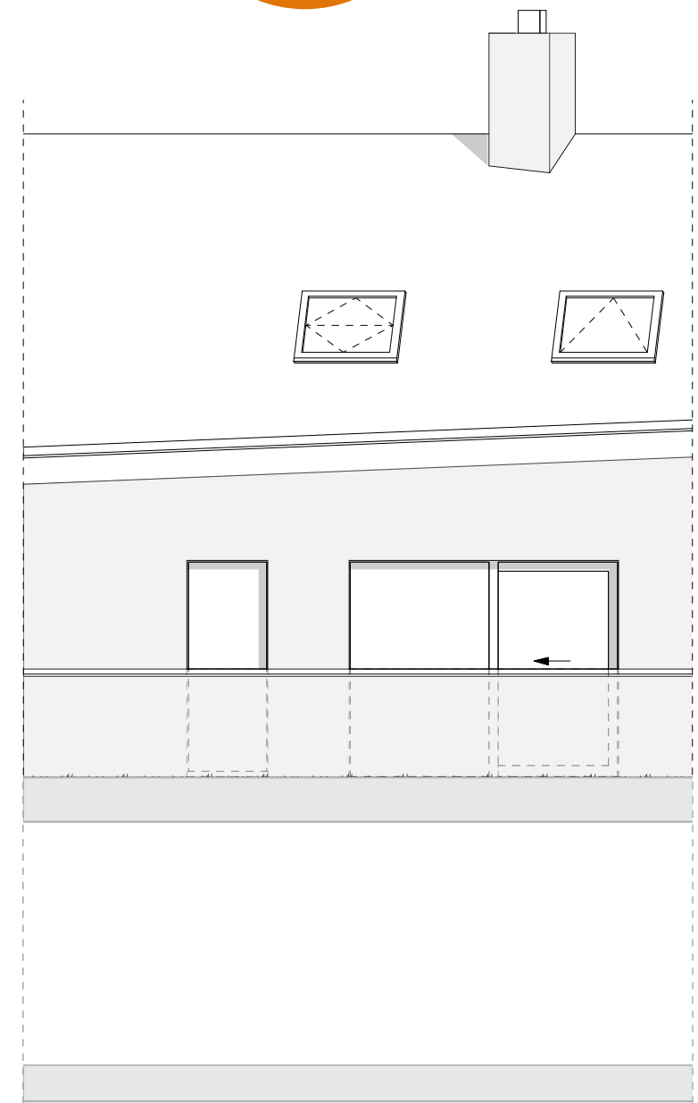
ACHTERGEVEL
